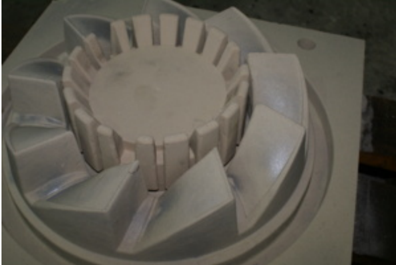
Lüfterrad Porsche 935
